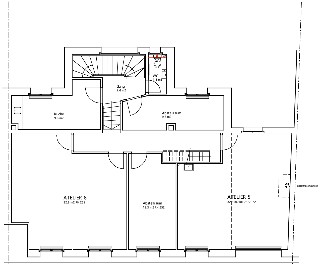
2. Obergeschoss
